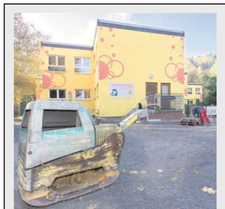
Gut gerüttelt: Per Rüttelplatte wird der Eingangsbereich glattgemacht und befestigt. Foto: Steffen Unger
